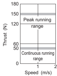
LM-U2PBB-07M-1SSO (*1)
