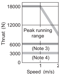
LM-FP5H-60M-1SS0 (*2)
